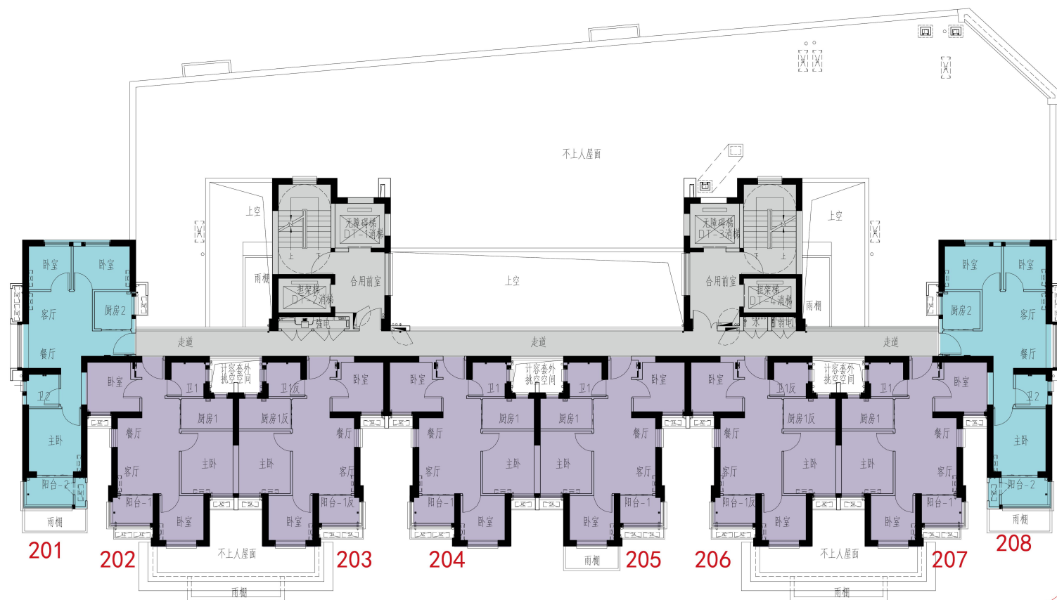
1#楼 二层平面图
